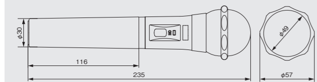
外形寸法図 [WM-P970/P902] (単位:mm)
