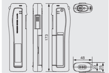
外形寸法図 [WM-P772] (単位:mm)
