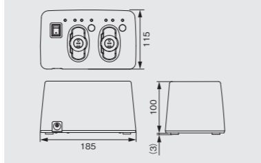
外形寸法図 (単位:mm)
