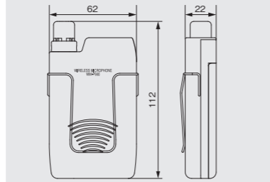
外形寸法図 [WM-P980] (単位:mm)
