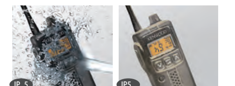
IP55 あらゆる方向からの噴流水による有害な影響が発生するほどの粉塵が中に入らない(防塵形)
