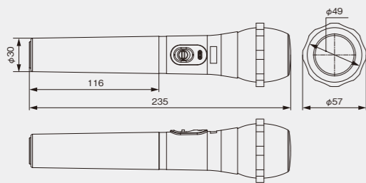
外形寸法図 [WM-P1070D] (単位: mm)
