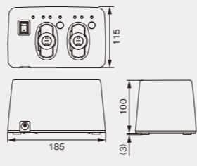
外形寸法図(単位: mm)
