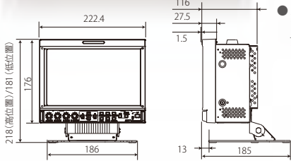
外観寸法図
