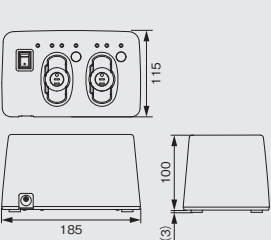
外形寸法図 (単位:mm)
