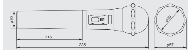
外形寸法図 [WM-P970/P902] (単位:mm)
