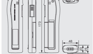
外形寸法図 [WM-P772] (単位:mm)
