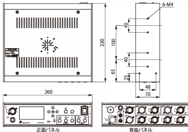
【ST#747BS 外観図】
