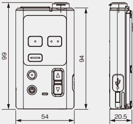
外形寸法図(単位:mm)
