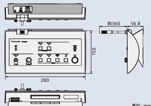
寸法図
