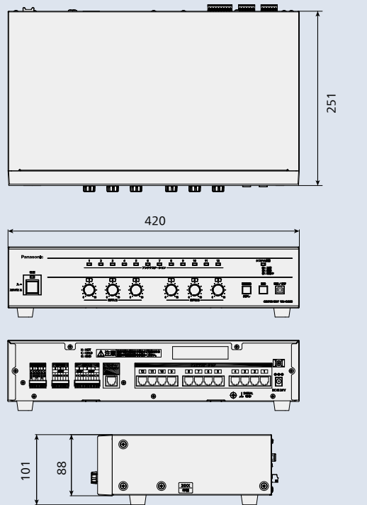
寸法図
