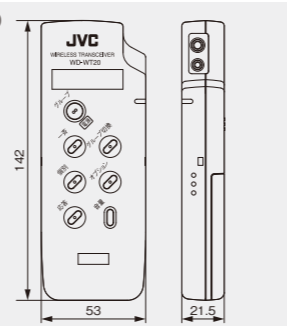
外形寸法図(単位:mm)
