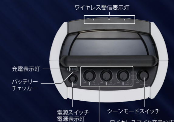
ワイヤレスの混信対策も万全 (WA-2800シリーズのみ) デジタルワイヤレスチューナー搭載可能 ※800MHz帯 B型ワイヤレス ワイヤレスユニット収納部 ワイヤレスチューナーユニット収納部 ワイヤレス接続端子 設定用ドライバー ライン出力端子 (外部アンプ等) 本体スピーカー入/切スイッチ 有線マイク音量つまみ 有線マイク入力端子 CD挿入口 USBメモリー挿入口 SDカード挿入口 クイック再生ボタン SD/USBプレーヤーユニット スピード調整つまみ 音程保持ボタン CDプレーヤーユニット スピード調整つまみ 外部入力音量つまみ 外部入力端子 (モノラル) (ポータブルCD、携帯音楽プレーヤーなど) 収納部 外部スピーカー音量つまみ 外部スピーカー端子 ニッケル水素充電電池収納部 電池ケース ニッケル水素充電電池端子
