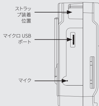
左側面図
