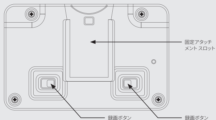
背面図
