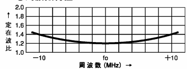
●周波数特性
