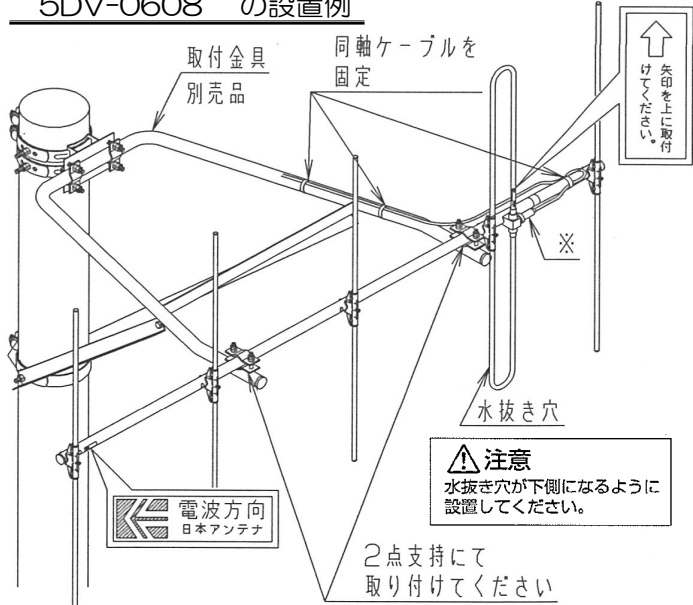
● 3DV-0608A 5DV-0608 の設置例
