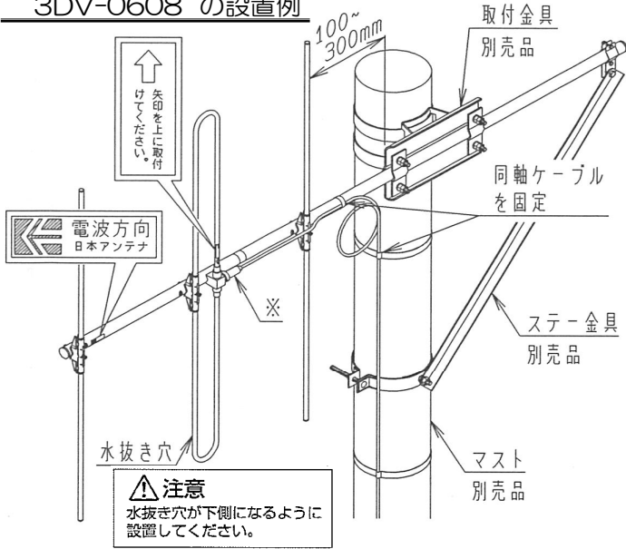
● 2DV-0608 3DV-0608 の設置例
