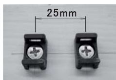
1. 25mm間隔に台座をビスで固定する
