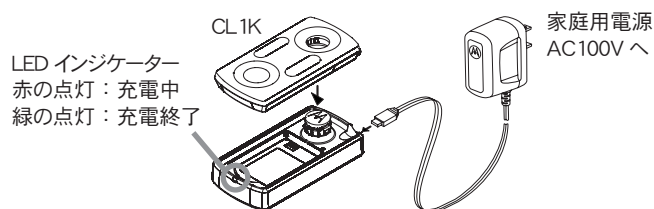
図 2：チャージースタンドと AC アダプターの接続
