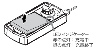
図 3：電池パックのみ充電する方法
