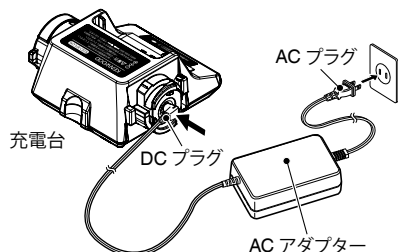
AC アダプター
