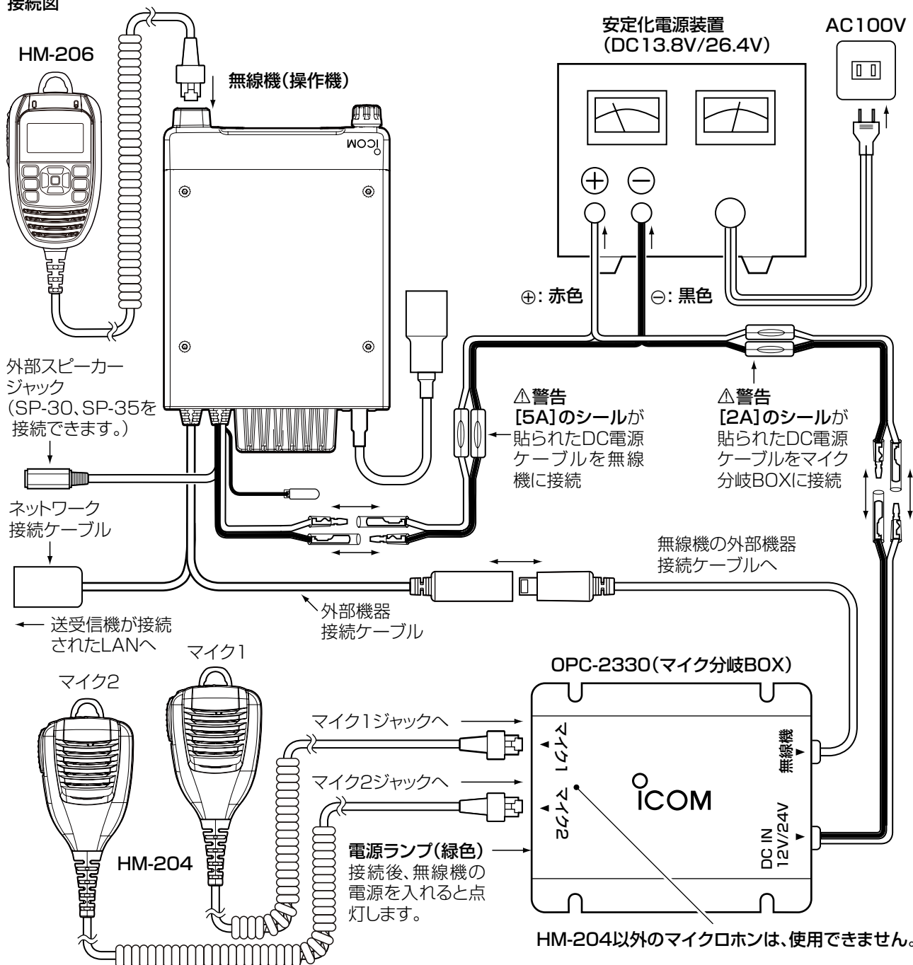
接続図
