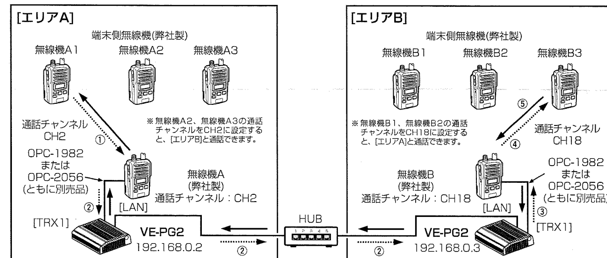
接続しているすべての無線機に送信 マルチキャストモードのイメージ図
