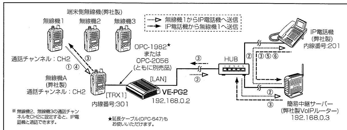
コンバーターモードの接続例
