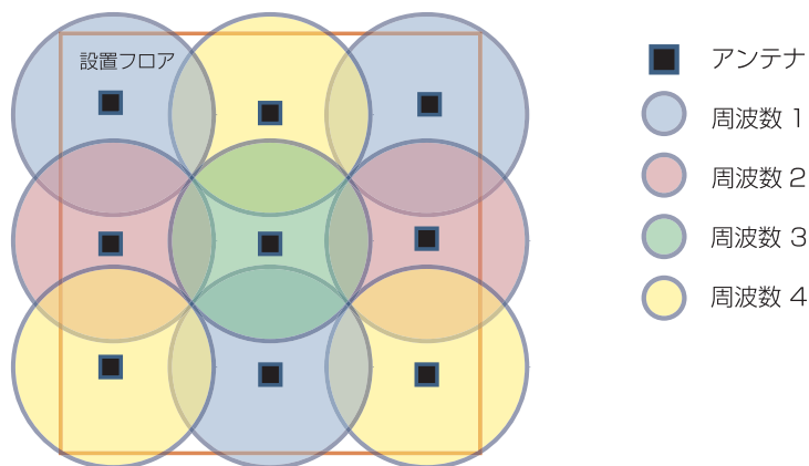
(混信を最初から考慮した 2.4GHz のアンテナ設置例)
