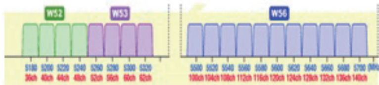
5GHz の周波数の分布
